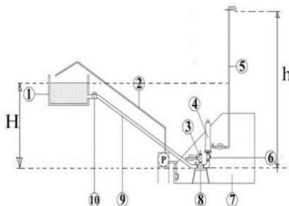
Gambar 1 Bagian - Bagian Pompa Hydram (Afif, 2016)
