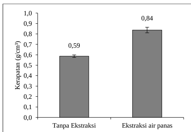
Gambar 2. Histogram kerapatan papan semen
