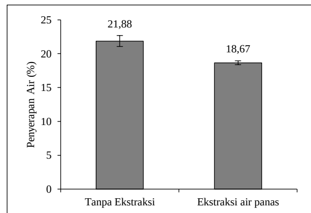
Gambar 3. Histogram penyerapan air papan semen
