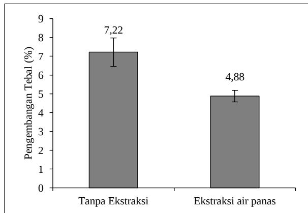
Gambar 4. Histogram pengembangan tebal papan semen
