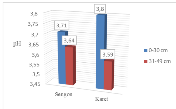
Gambar 1. pH Tanah
