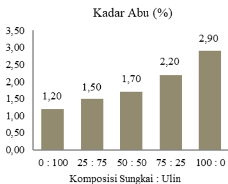
Gambar 5. Kadar Abu Briket Arang Sungkai dan Ulin
