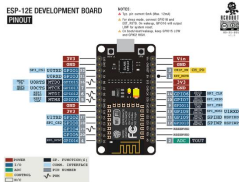
Gambar 4. ESP-8266 NodeMCU
