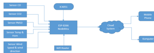
Gambar 11. Desain Arsitektur Sistem
