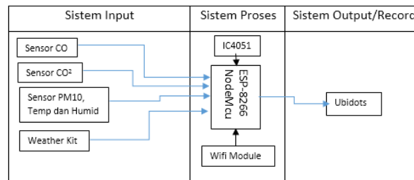
Gambar 13. Cara kerja alat
