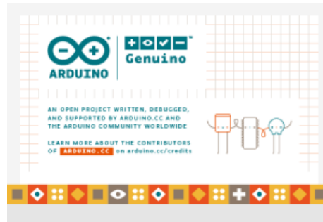
Gambar 5. Arduino IDE
