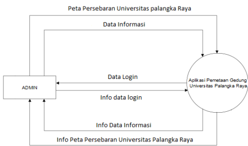
Gambar 4.1 DFD Level 1
