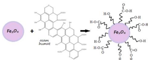
Gambar 4. Ilustrasi pengikatan asam humat dengan Fe 3 O 4 dalam AH-Fe 3 O 4 [8]
