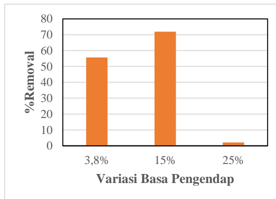
Gambar 7. Pengaruh variasi basa pengendap dari AH- \text{Fe}_3\text{O}_4 terhadap daya adsorpsi congo red
