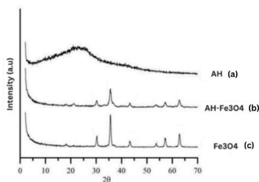
Gambar 5. Diffraktogram XRD dari asam humat (a), AH-Fe 3 O 4 (b) dan Fe 3 O 4 (JCPDS 19-0629) (c)
