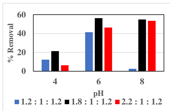
Gambar 6. Grafik perbandingan rasio asam humat : \text{Fe}^{2+} : \text{Fe}^{3+} terhadap daya adsorpsi congo red pada rentang pH 4, 6 dan 8
