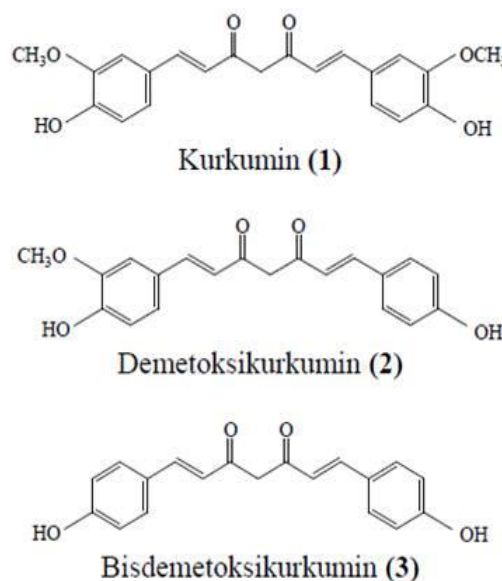
Gambar 1. Struktur senyawa kurkumin, demetoksikurkumin dan bisdemetoksi kurkumin
