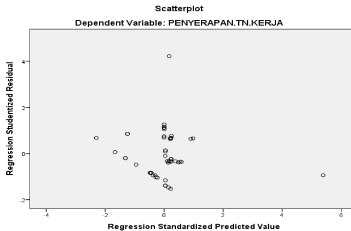
Gambar 4.1 Uji Heterokedastisitas
